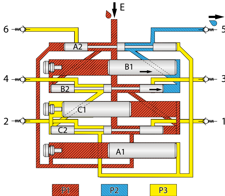
Abb.15 Schmierstoffverlauf am Beispiel eines SSVD-6 Verteilers Phase 7 und 8
