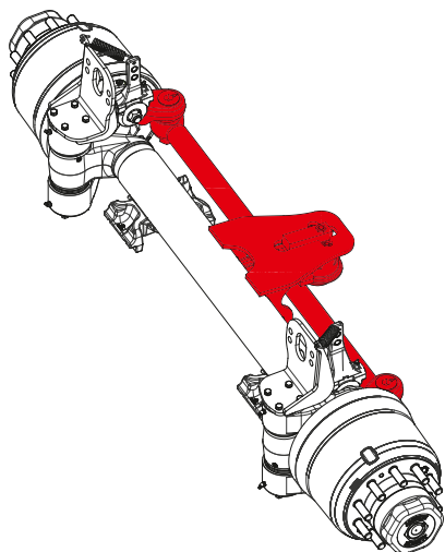
Nachlaufenkachsen (NL) mit Spurstange, Stabilisierungs- und Verriegelungseinheit
