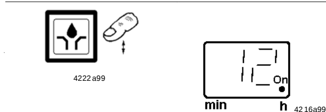
Abb. 12-3 Änderung der Pausenzeit "P1" (Stunden)
