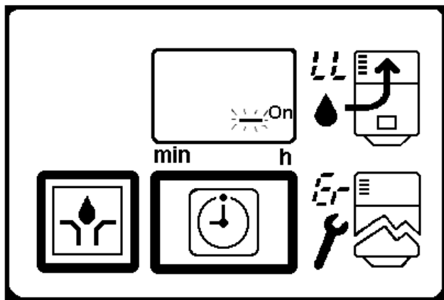
Abb. 10-1 Folientastatur
