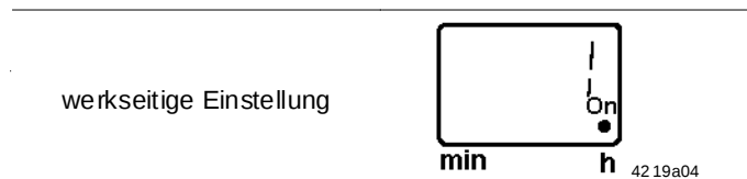
Abb. 12-8 Werkseitige Einstellung der Verteilerumläufe je Arbeitszyklus "P3"
