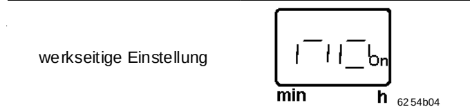
Abb. 12-11 Werkseitige Einstellung des Ausgangssignals "P4"
