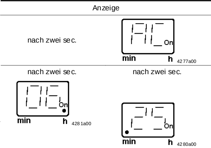
Abb. 13-6 Anzeige automatisch ausgelöster Arbeitszyklen
