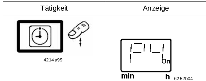
Abb. 12-10 Wechsel zum Ausgangssignal "P4" (nc oder no)
