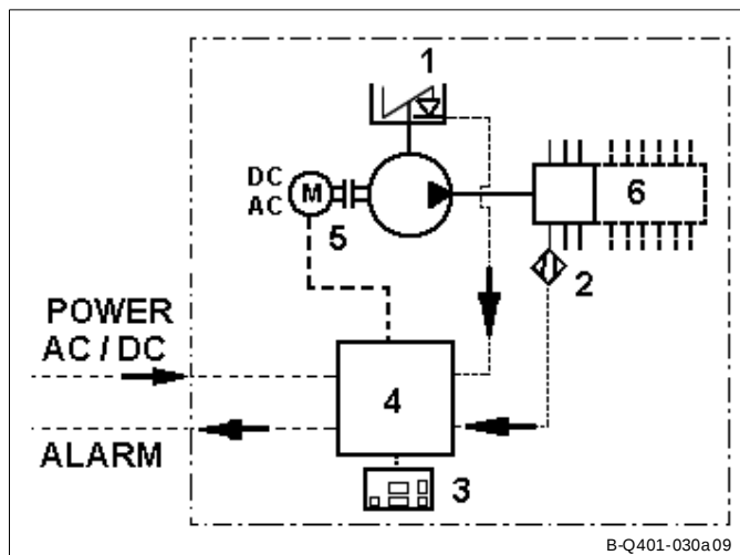
Abb. 7-1 QLS-Schema
