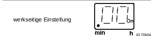
Abb. 12-5 Werkseitige Einstellung der Pausenzeit "P2" (Minuten)
