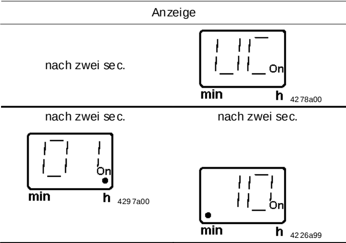
Abb. 13-7 Anzeige manuell ausgelöster Zusatzschmierungen
